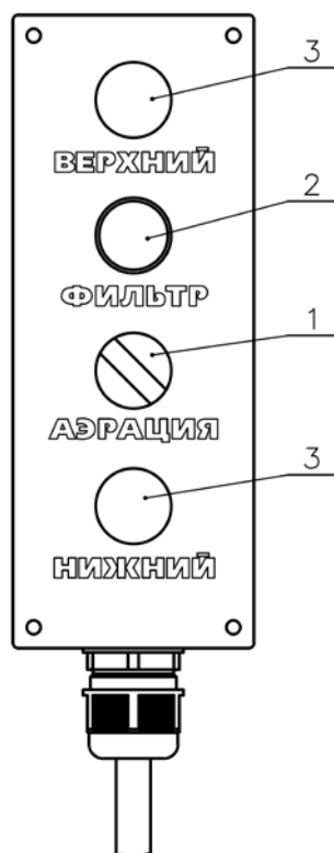
Рис.6. Пульт выносной
